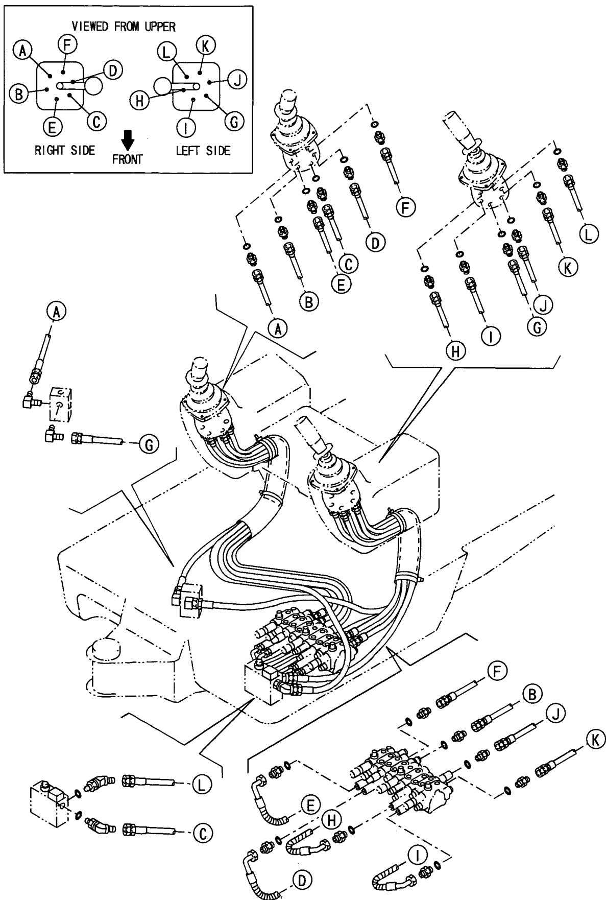
Fig. 51 油圧配管(ダイレクト) HYD. OIL PIPING(DIRECT)
