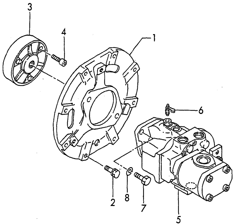
Fig. 29 油圧ポンプ & 軸継手 HYD. OIL PUMP & JOINT
