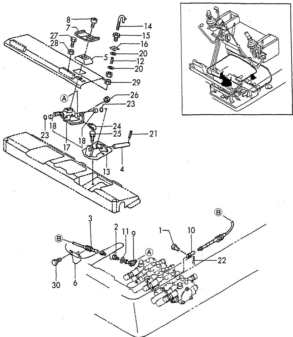
Fig. 21 操縦装置(PTO) CONTROL EQUIPMENT(P. T. O.)
