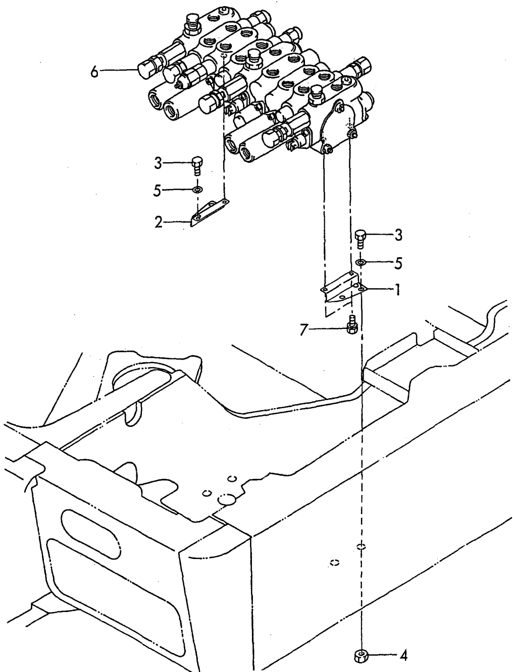
Fig. 38 コントロールバルブ CONTROL VALVE
