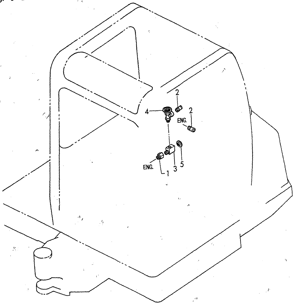
ig. 13 ヒーター HEATER
