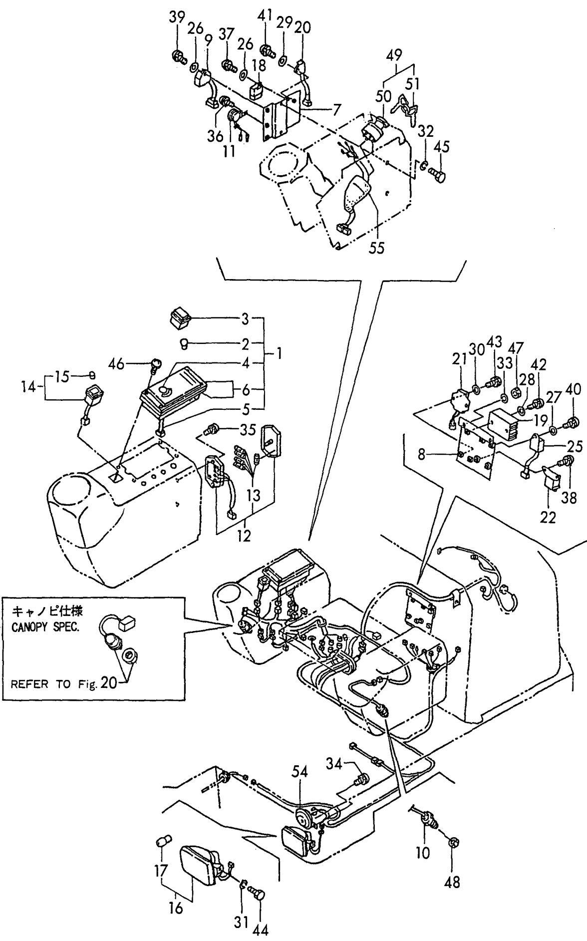
Fig. 10 電装品(機器:キャビン, キャノピー共通) ELECTRIC PART (EQUIPMENT: CABIN, CANOPY)
